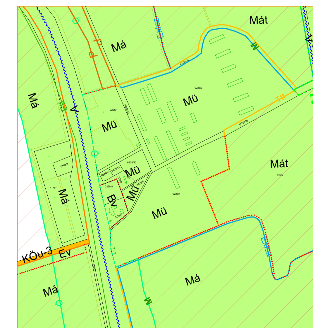
ÁLLAMPUSZTA MIKLA M=1:5000
