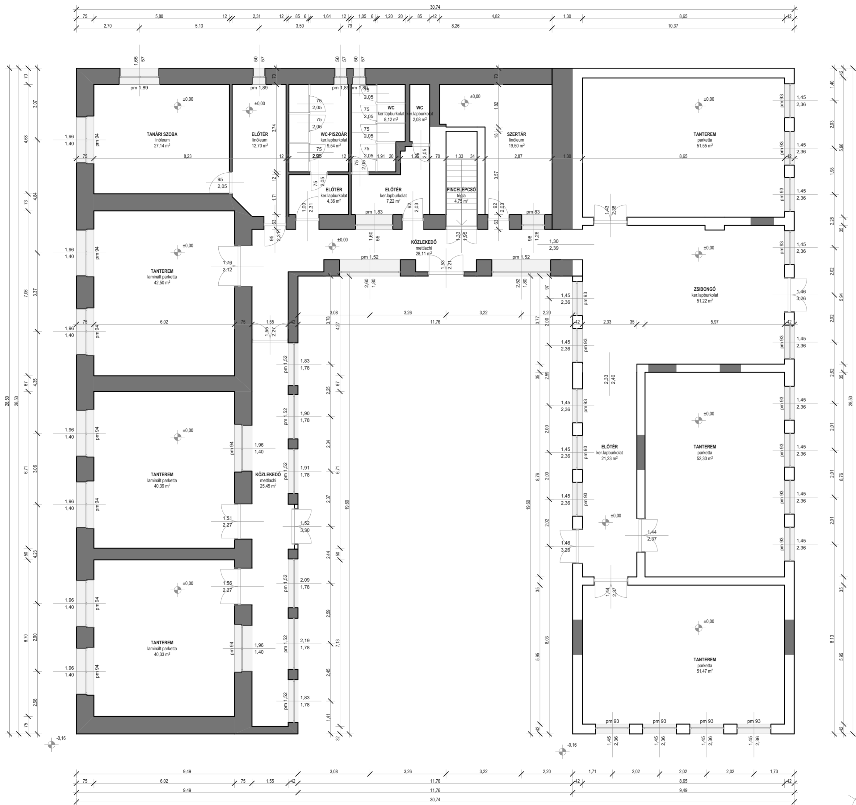
ÁLLAPOT FÖLDSZINT ALAPRAJZ M=1:100
